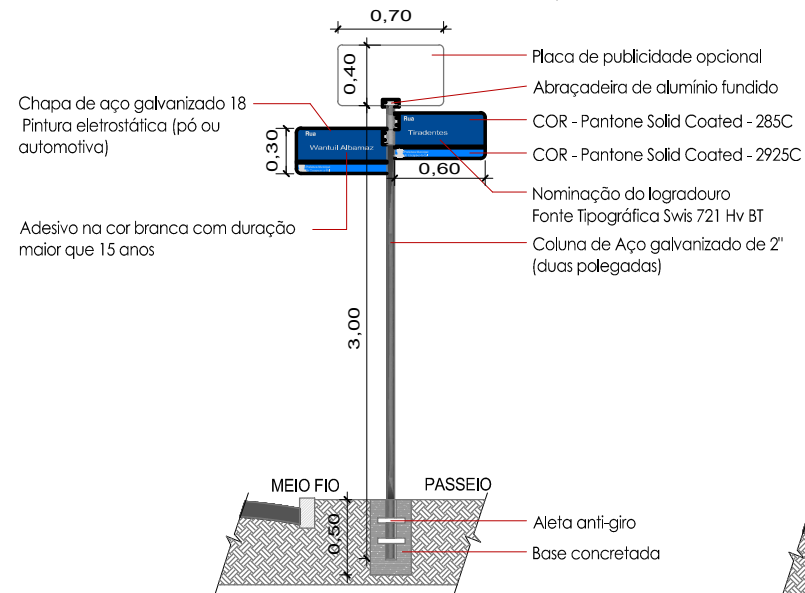
Detalhe 1 - Placa de esquina
