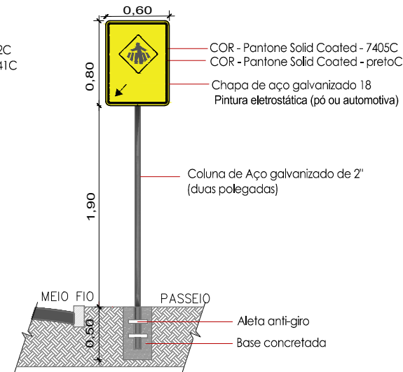
Detalhe 4 - Placa (A-32b) passagem sinalizada de pedestres
