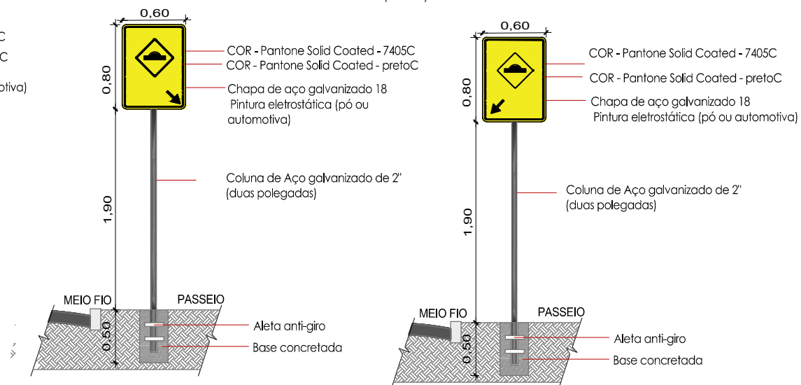
Detalhe 5 - Placa (A-18) lombada
