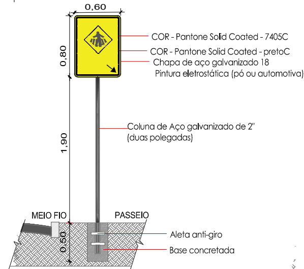
Detalhe 4 - Placa (A-32b) passagem sinalizada de pedestres
