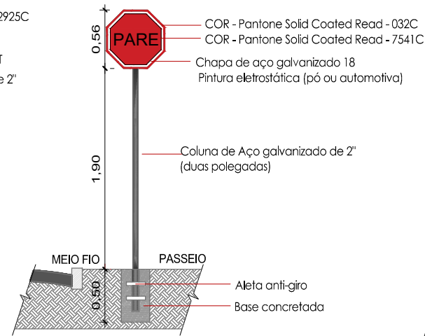
Detalhe 2 - Placa (R-1) parada obrigatória
