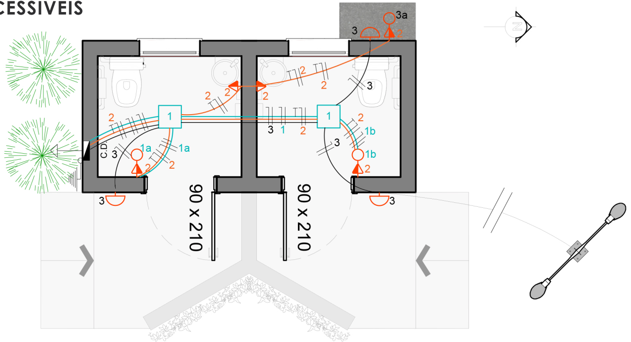
PLANTA BAIXA - ELÉTRICA ESC.: 1/50
