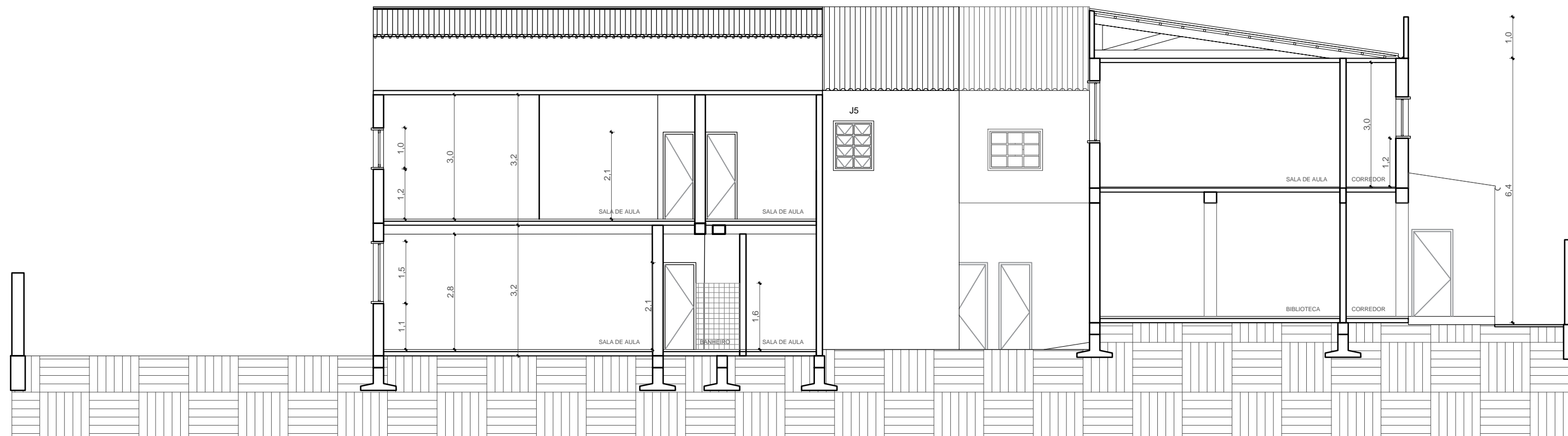
1 CORTE C C' ESCALA 1/100
