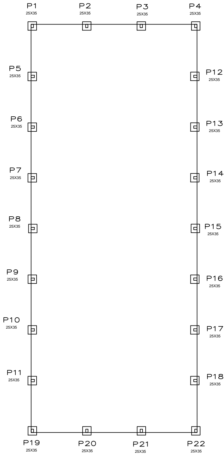
PLANTA DE LOCALIZAÇÃO DAS FUNDAÇÕES e PILARES
