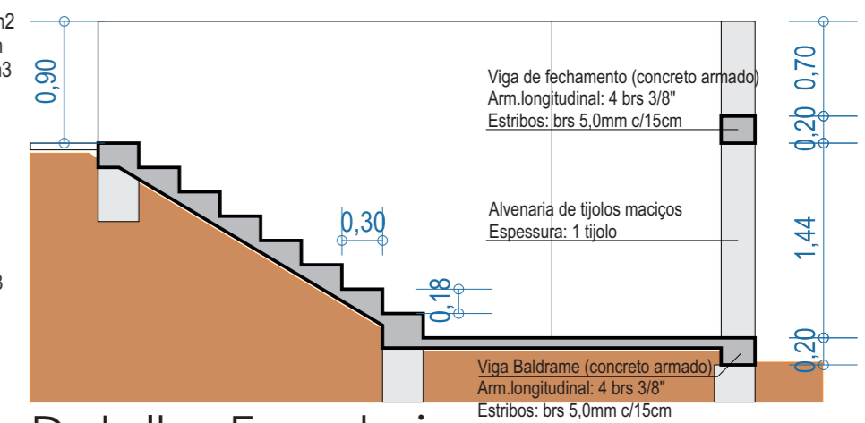
Detalhe Escadaria esc: 1:50
