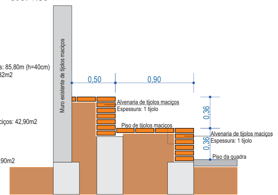
Detalhe Arquibancadas esc: 1:25
