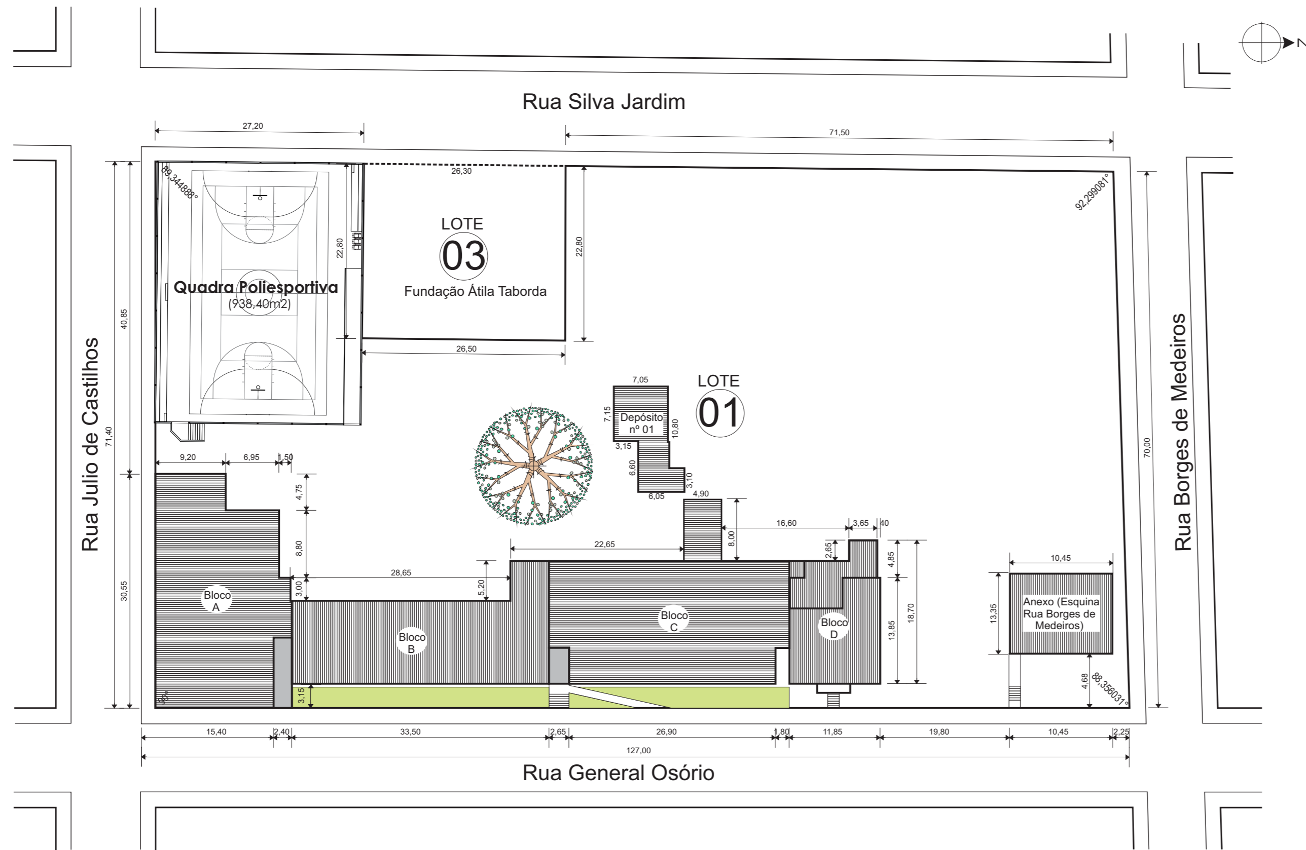
Situação e Localização - Escala: 1/250
