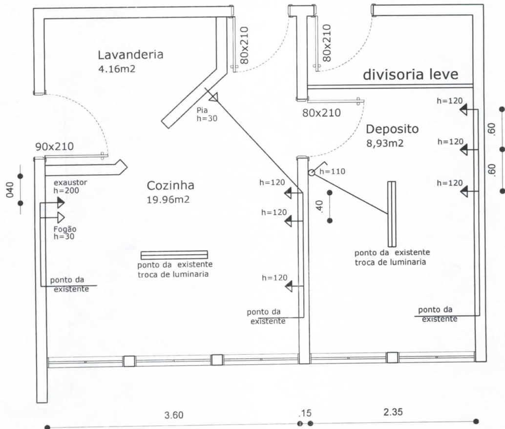
PLANTA ELETRICA
