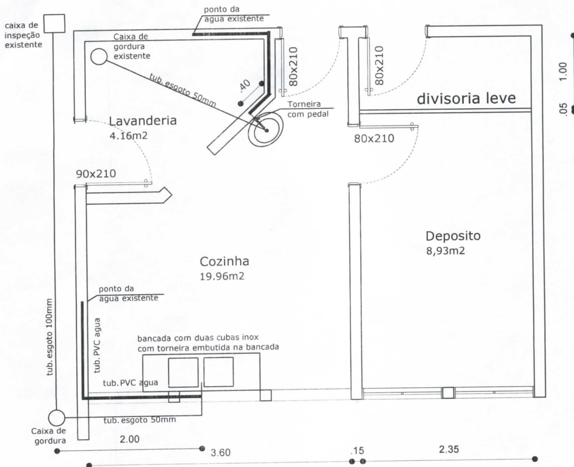
PLANTA HIDRAULICA
