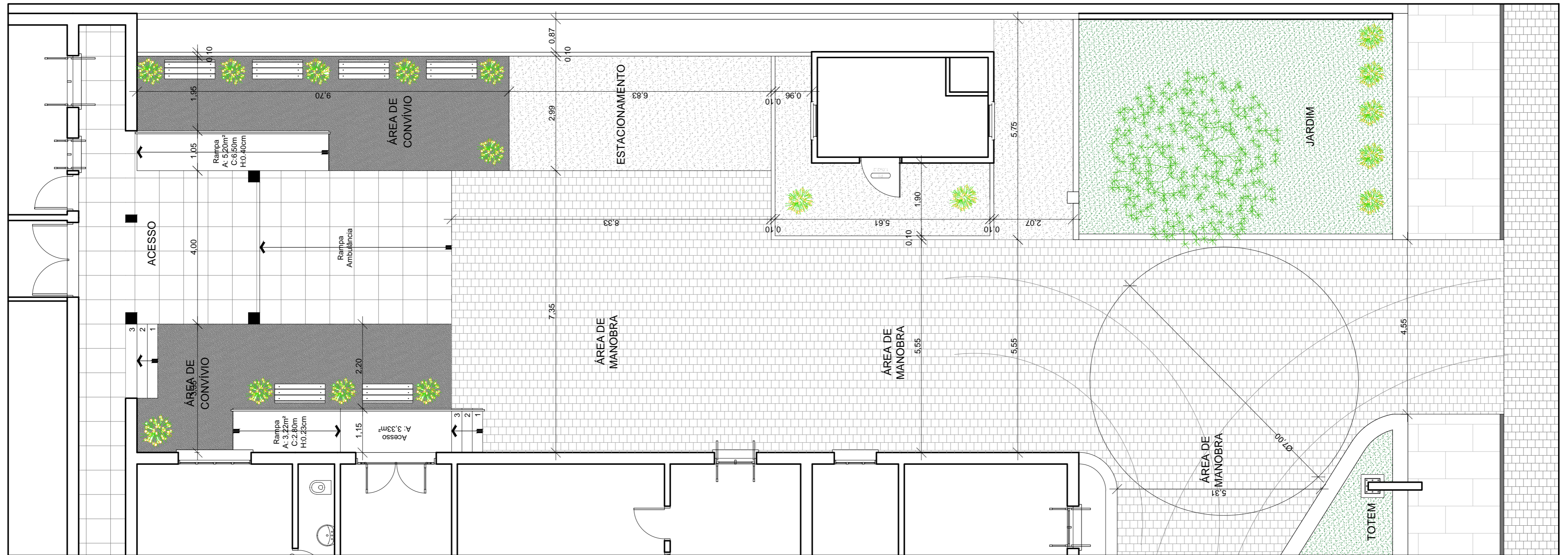
PLANTA BAIXA - TÉCNICA ESCALA: 1:75
