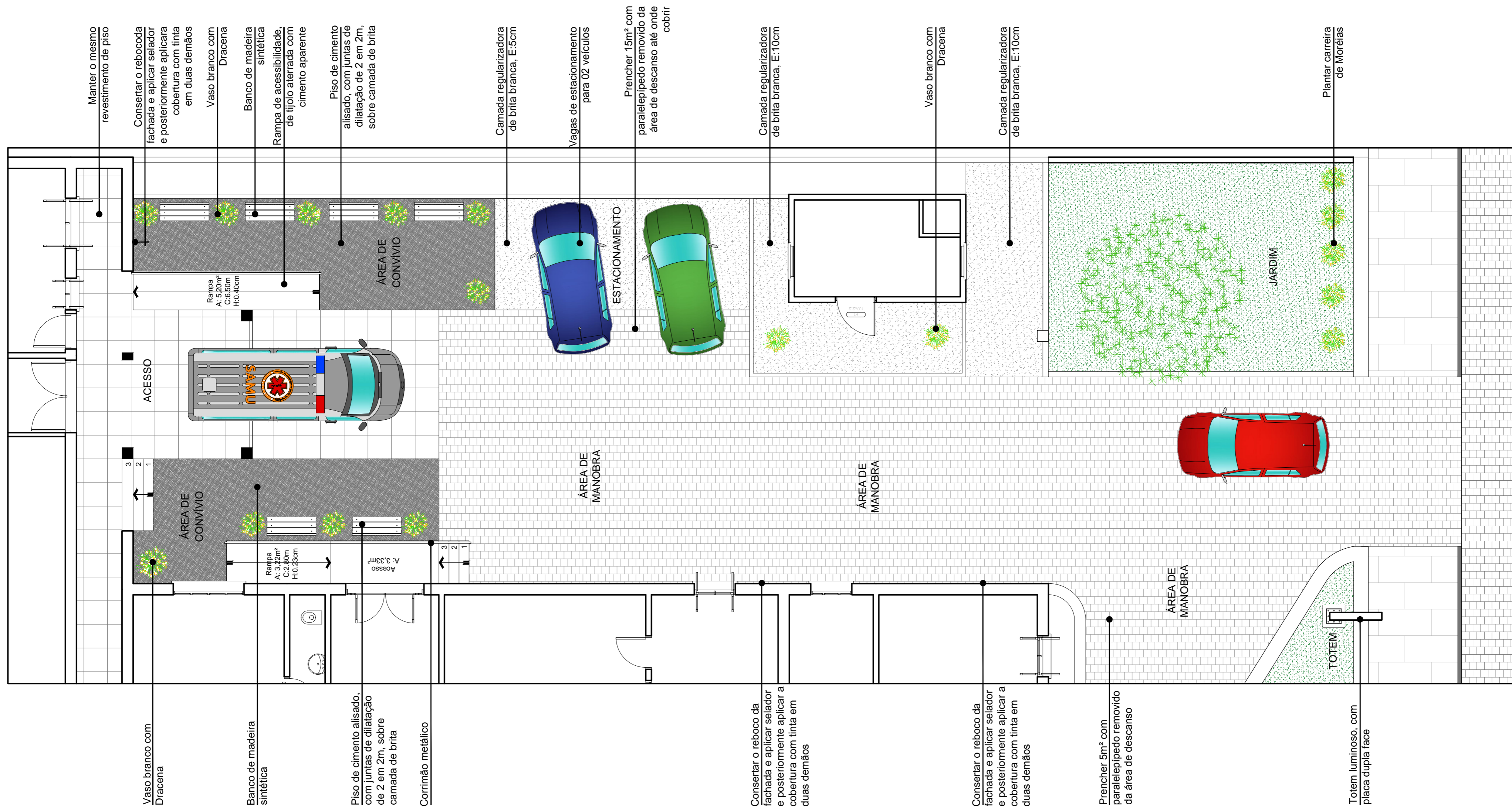
PLANTA BAIXA - LAYOUT ESCALA: 1:75
