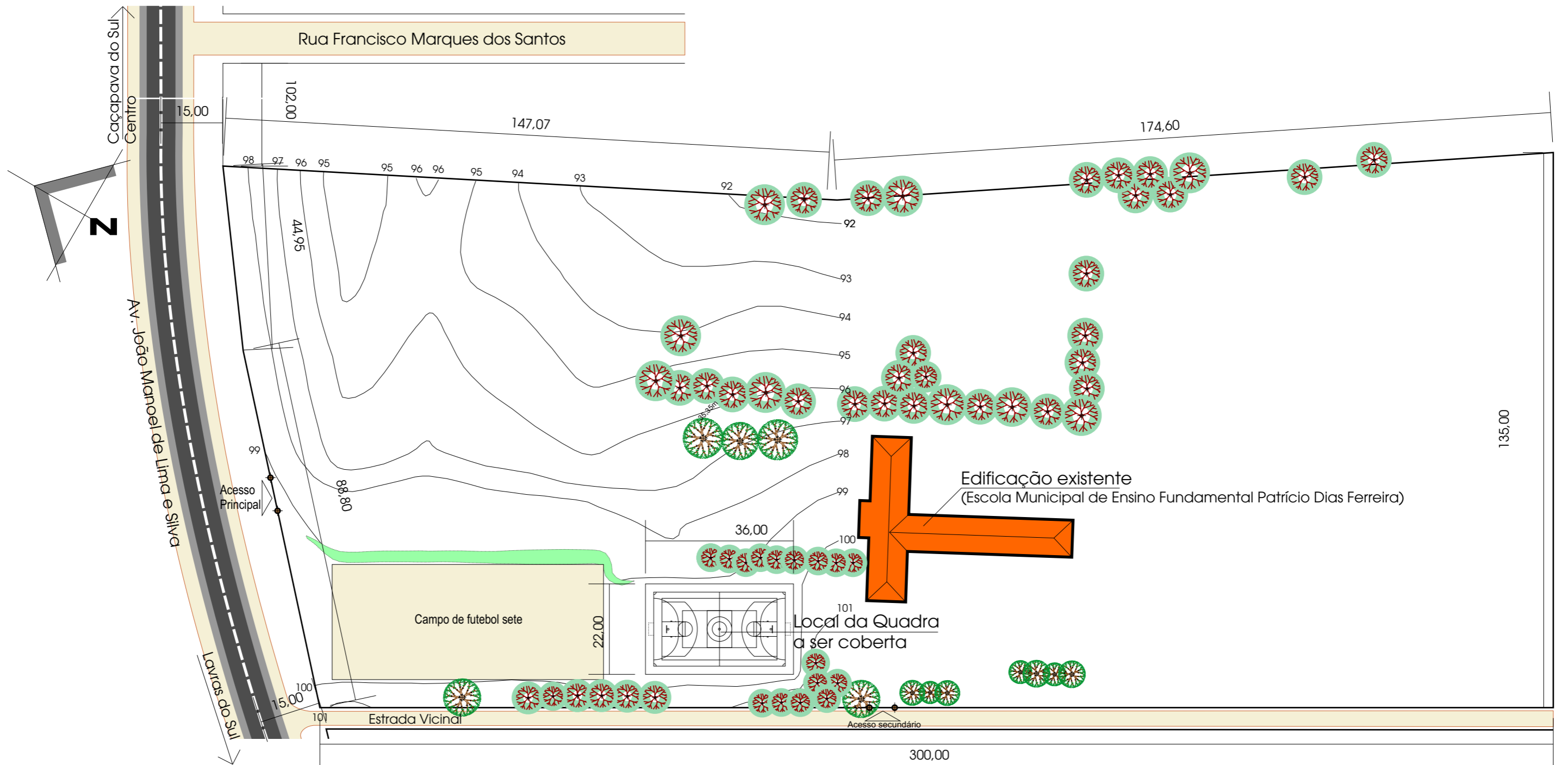
Planta de Situação e Localização esc: 1:1000
