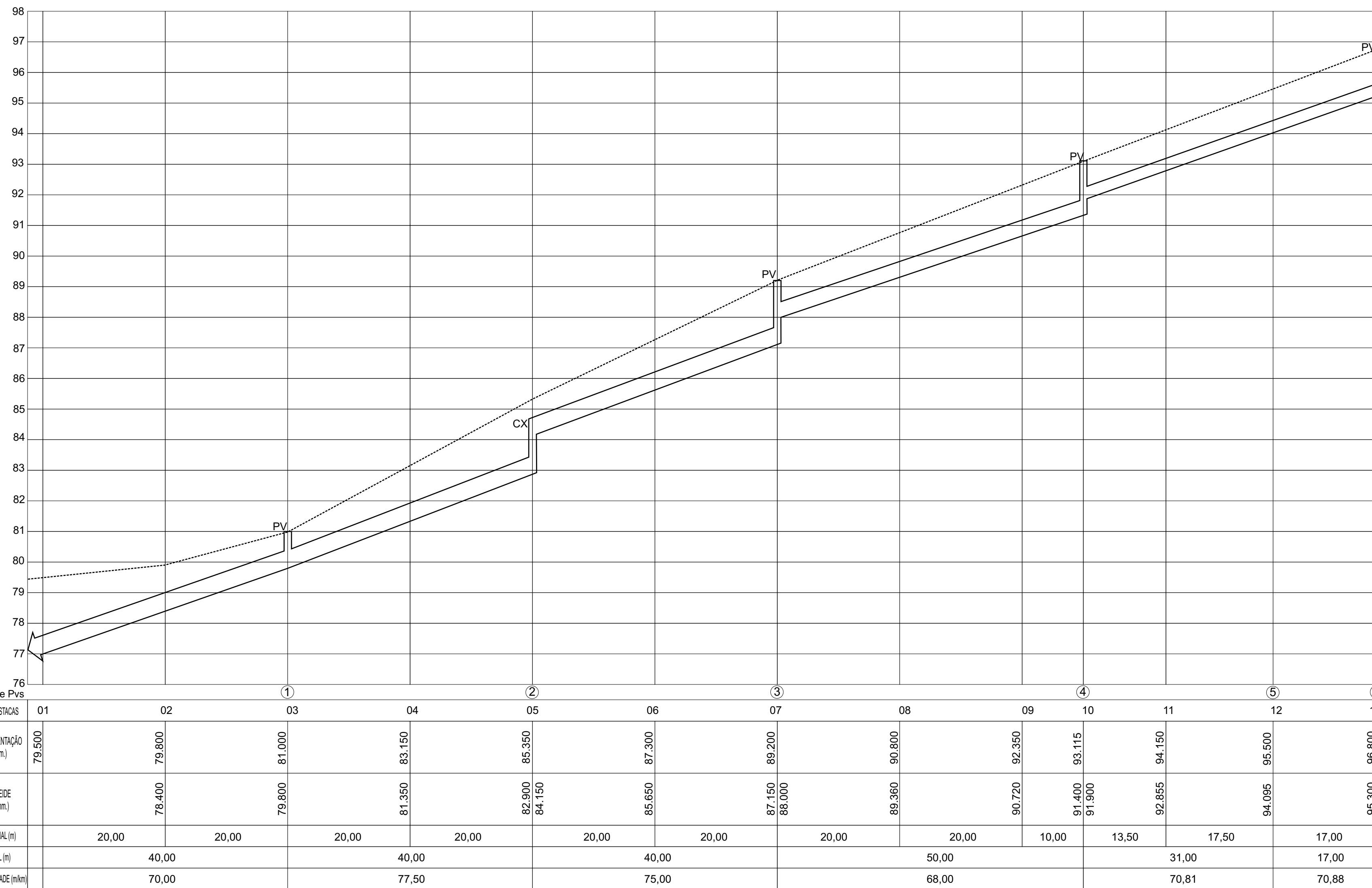
PERFIL LONGITUDINAL esc. vertical: 1:100 esc. horizontal: 1:500
