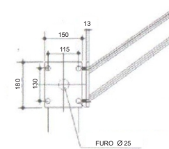
DETALHE DA CAIXA VISTA LATERAL
