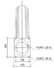
DETALHE DA FLANGE VISTA POSTERIOR
