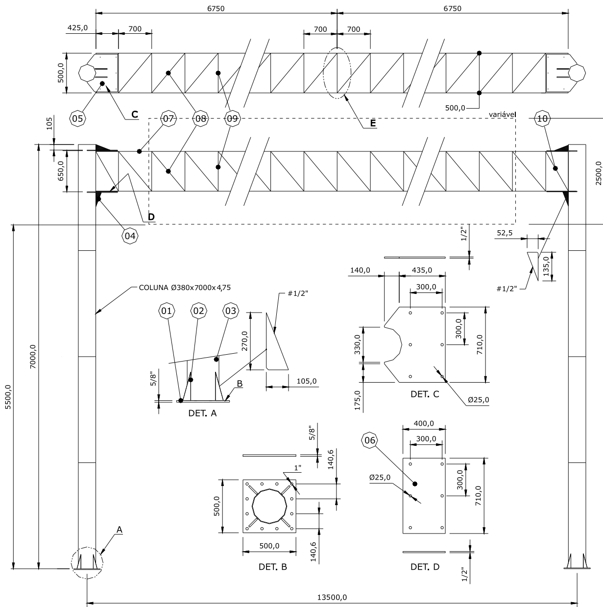
Pórtico Treliçado
