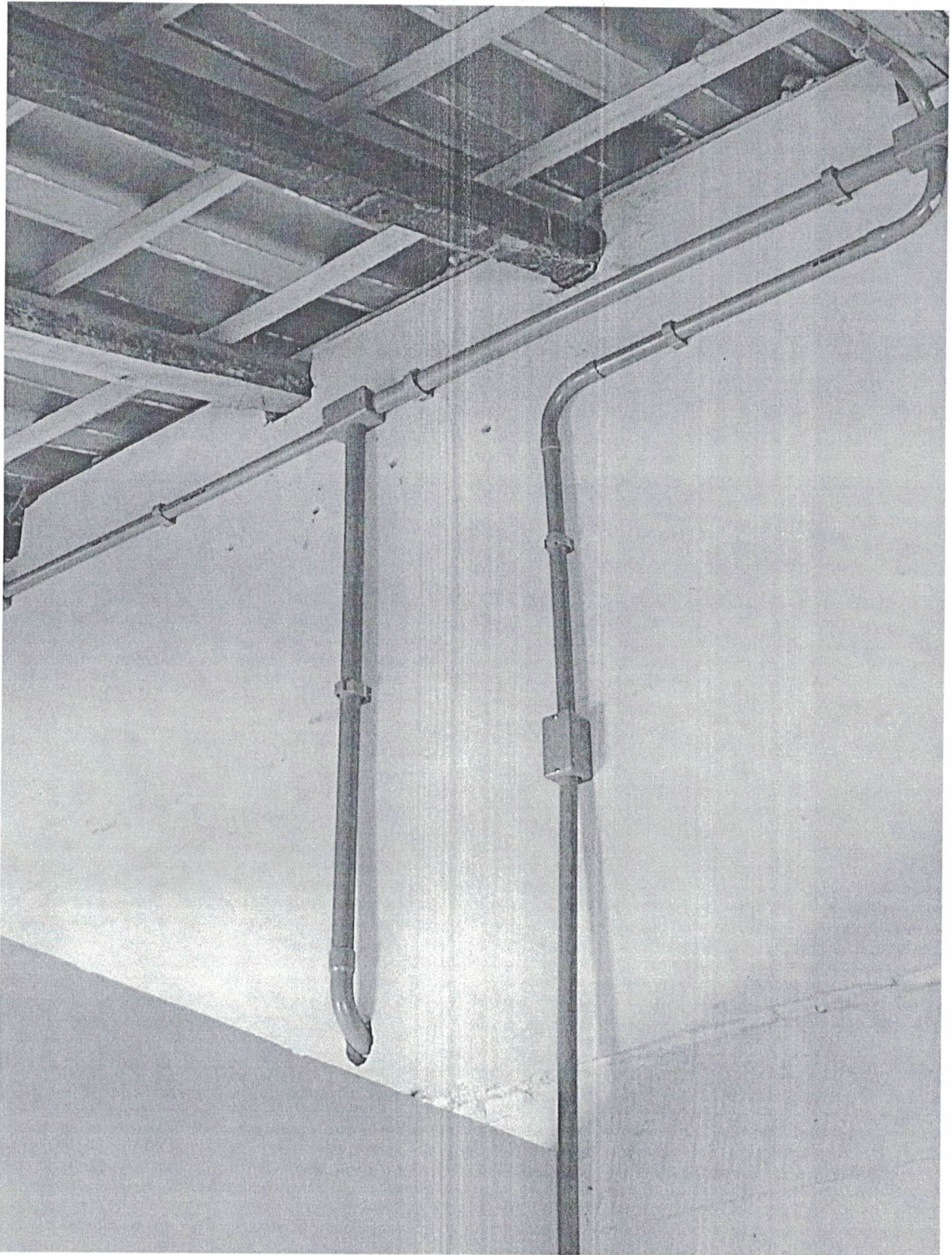
Foto 4: Rede elétrica feita por condutores, conforme orientação dos Bombeiros.
