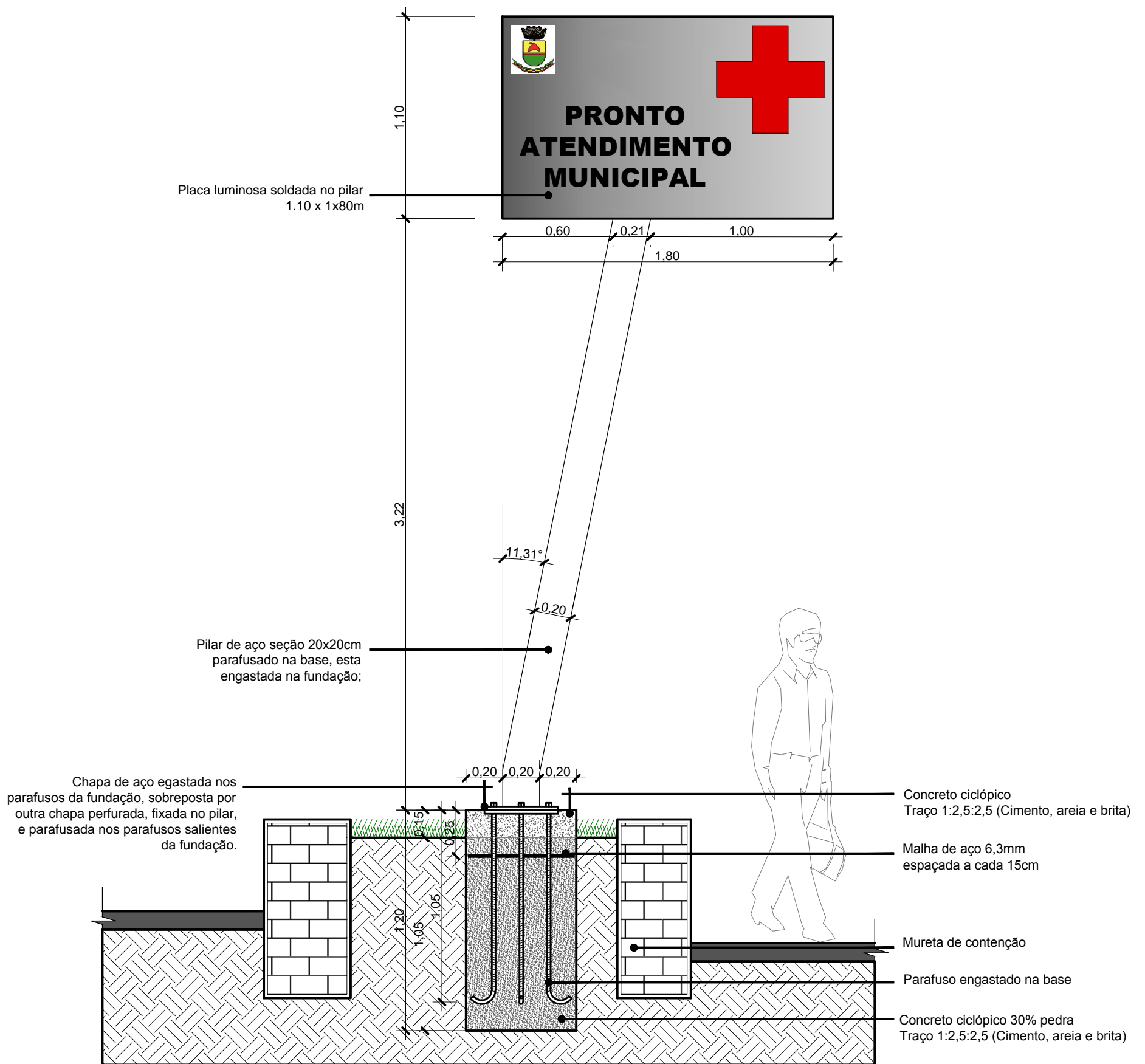
PLACA LUMINOSA ELEVÇÃO ESCALA: 1:25
