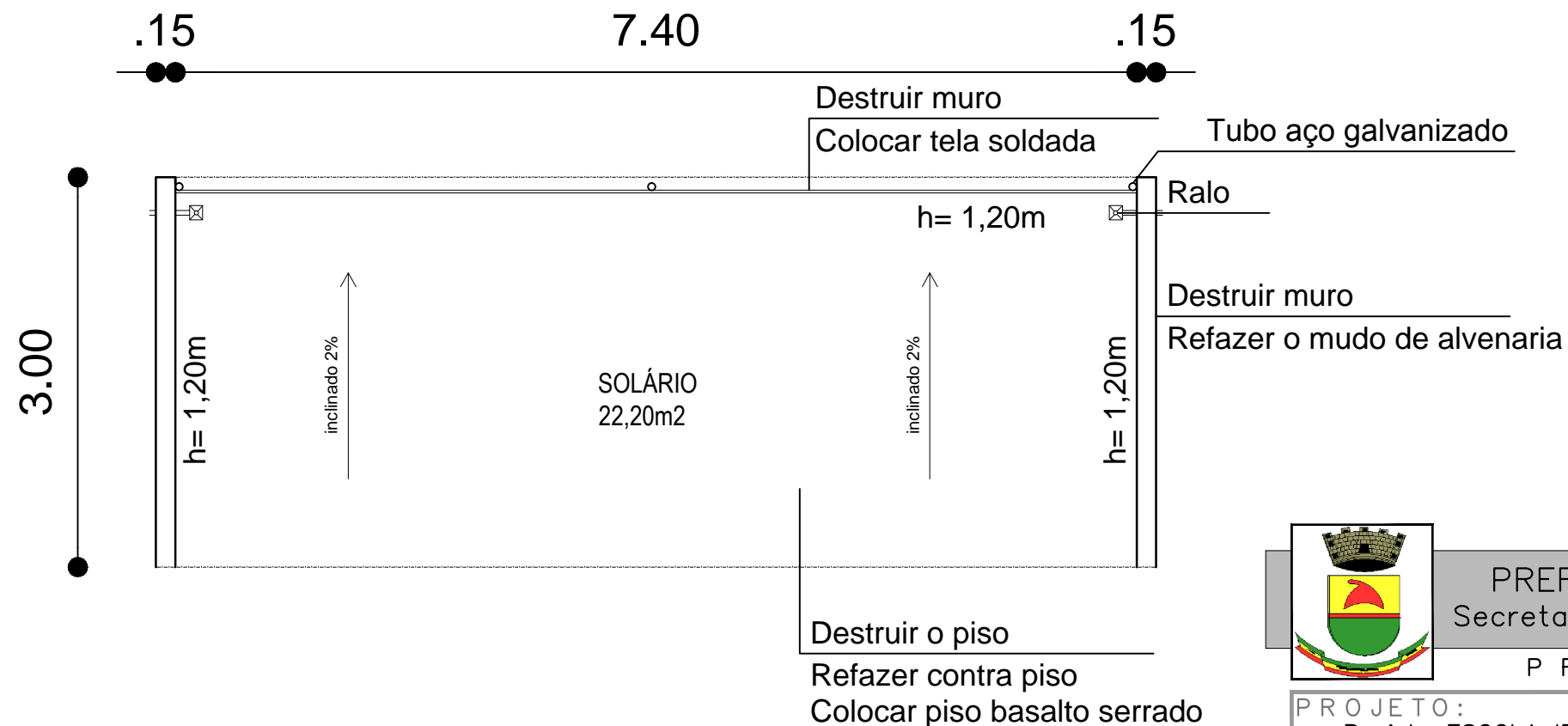
02 PLANTA BAIXA escala: 1/50
